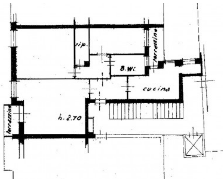
Planimetria
